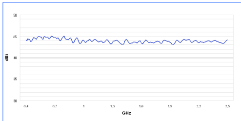
게인 그래프 HyperLOG 4025X
