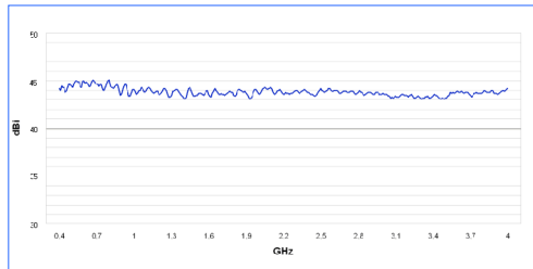
게인 그래프 HyperLOG 4040X
