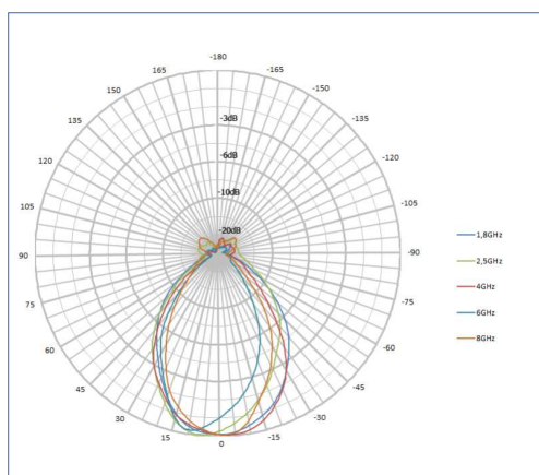
수평 패턴 HyperLOG 40 X 시리즈
