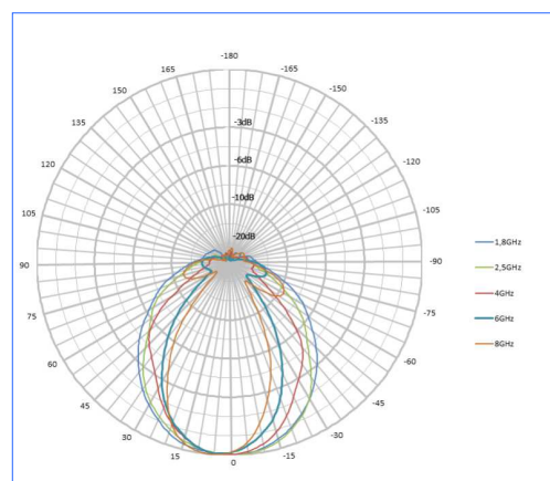
수직 패턴 HyperLOG 40 X 시리즈
