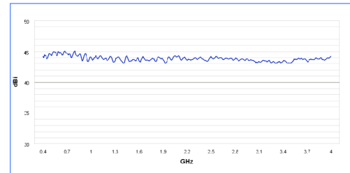
게인 그래프 HyperLOG 4060X
