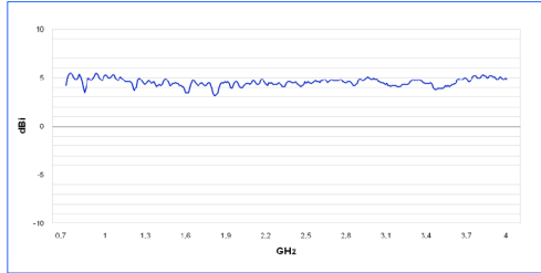
이득 그래프 HyperLOG 7040
