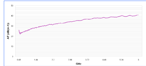
안테나 인수 HyperLOG 7060
