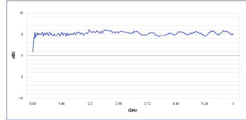
이득 그래프 HyperLOG 7060
