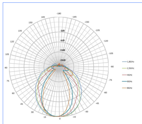
수직 패턴 HyperLOG 70xx 시리즈
