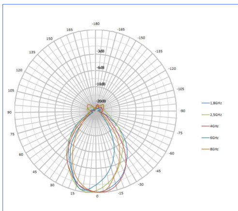
수평 패턴 HyperLOG 70xx 시리즈
