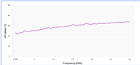
안테나 인수 HyperLOG 7025
