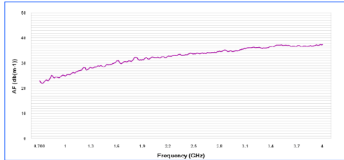
안테나 인수 HyperLOG 7040
