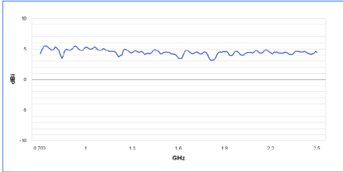
이득 그래프 HyperLOG 7025
