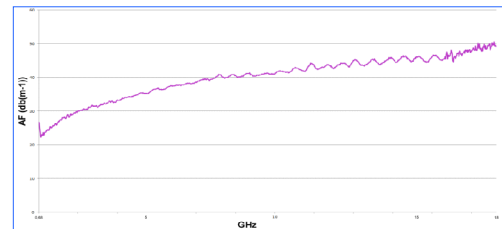
안테나 인수 HyperLOG 60180
