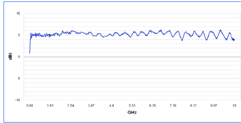
이득 그래프 HyperLOG 60100
