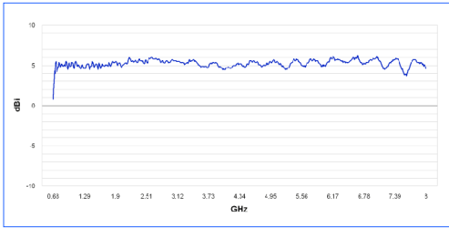
이득 그래프 HyperLOG 6080
