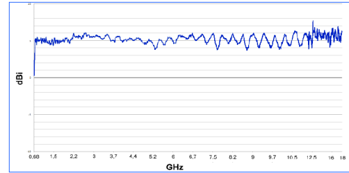
이득 그래프 HyperLOG 60180
