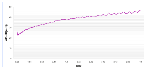
안테나 인수 HyperLOG 60100
