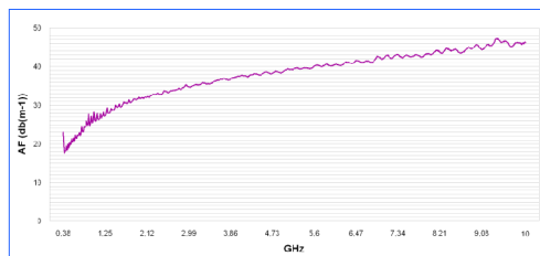
안테나 인수 HyperLOG 30100
