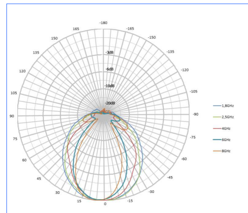
수직 패턴 HyperLOG 30xx Serie
