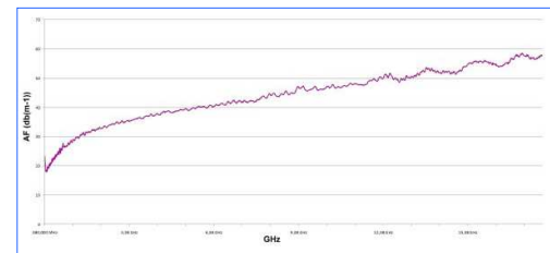
안테나 인수 HyperLOG 30180
