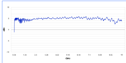
이득 그래프 HyperLOG 30100
