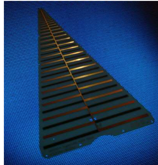
금 코팅, 보호용 TEFLON 정밀 안테나
