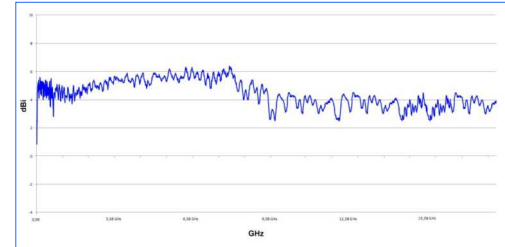
이득 그래프 HyperLOG 30180
